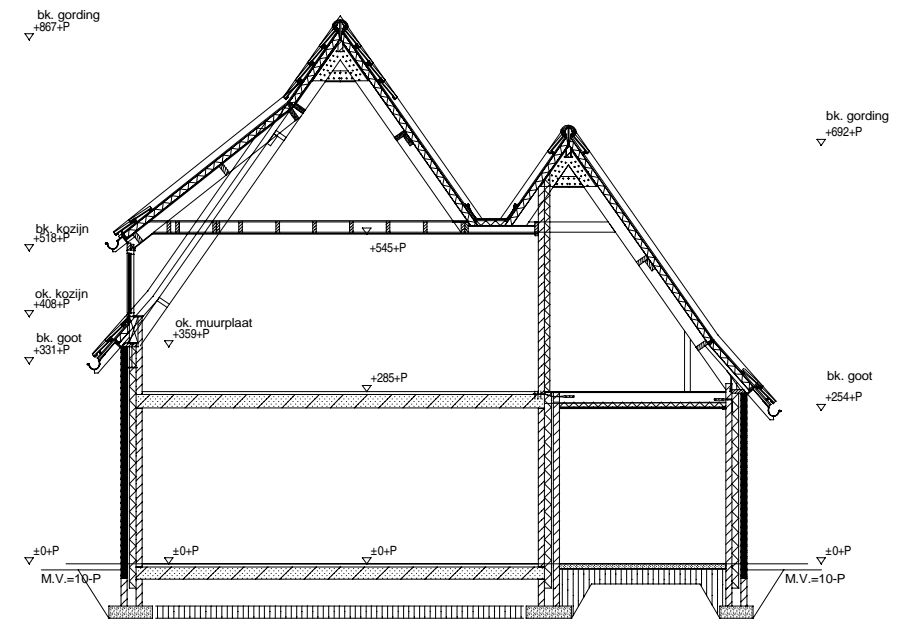
DOORSNEDE
