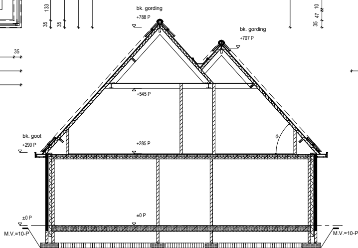
DOORSNEDE
